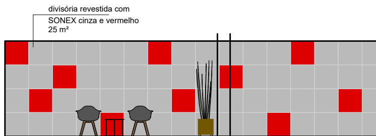
VISTA 3 esc 1/100
