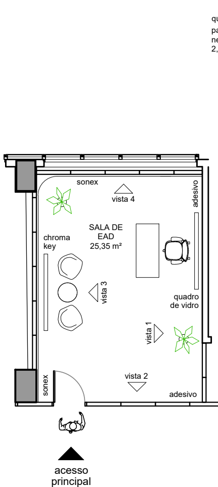
LAYOUT SALA EAD_proposta esc 1/100
