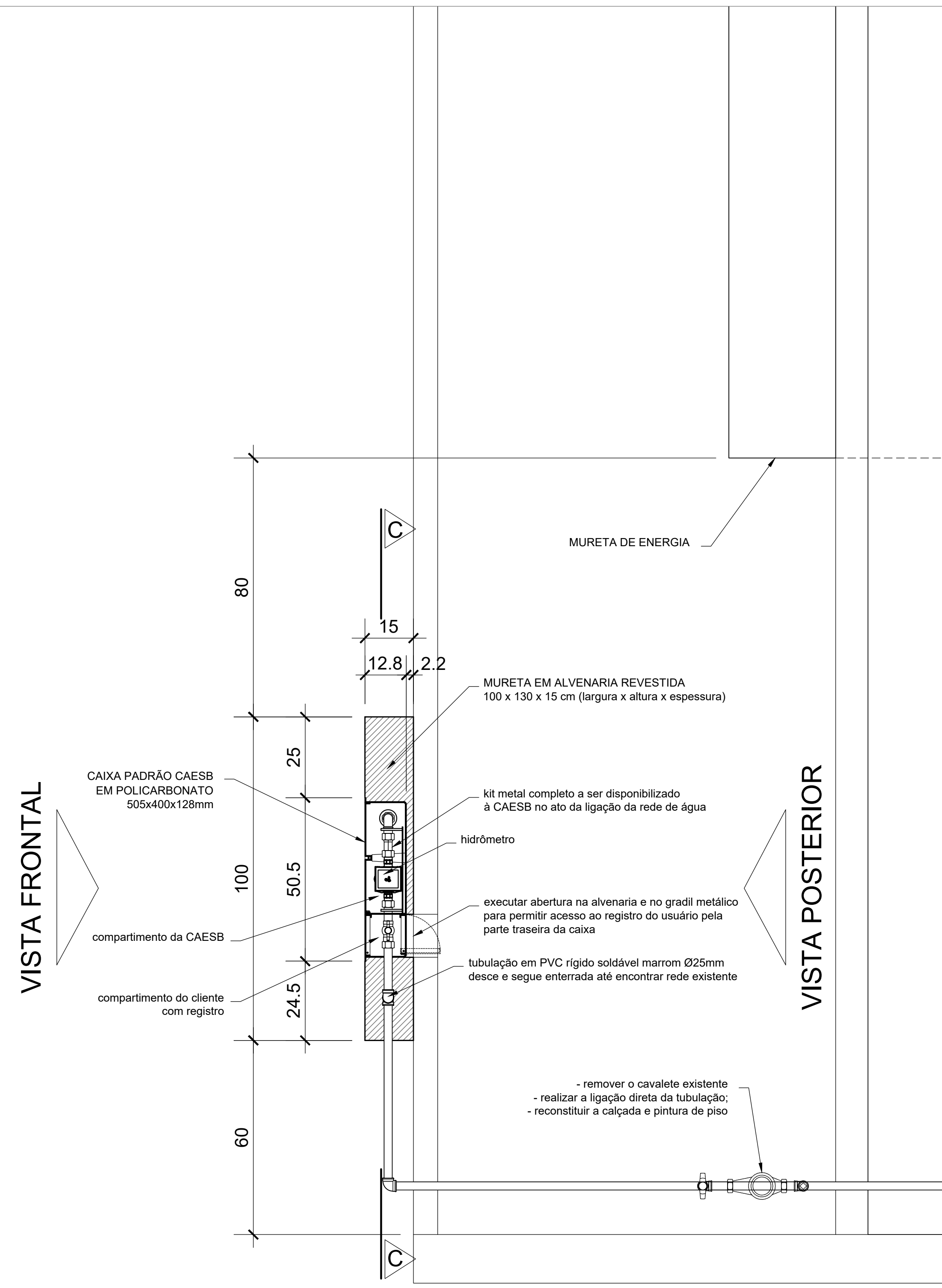
DETALHE DA INSTALAÇÃO DE HIDRÔMETRO PADRÃO CAESB EM ABRIGO (MURETA) ESCALA:1/10
