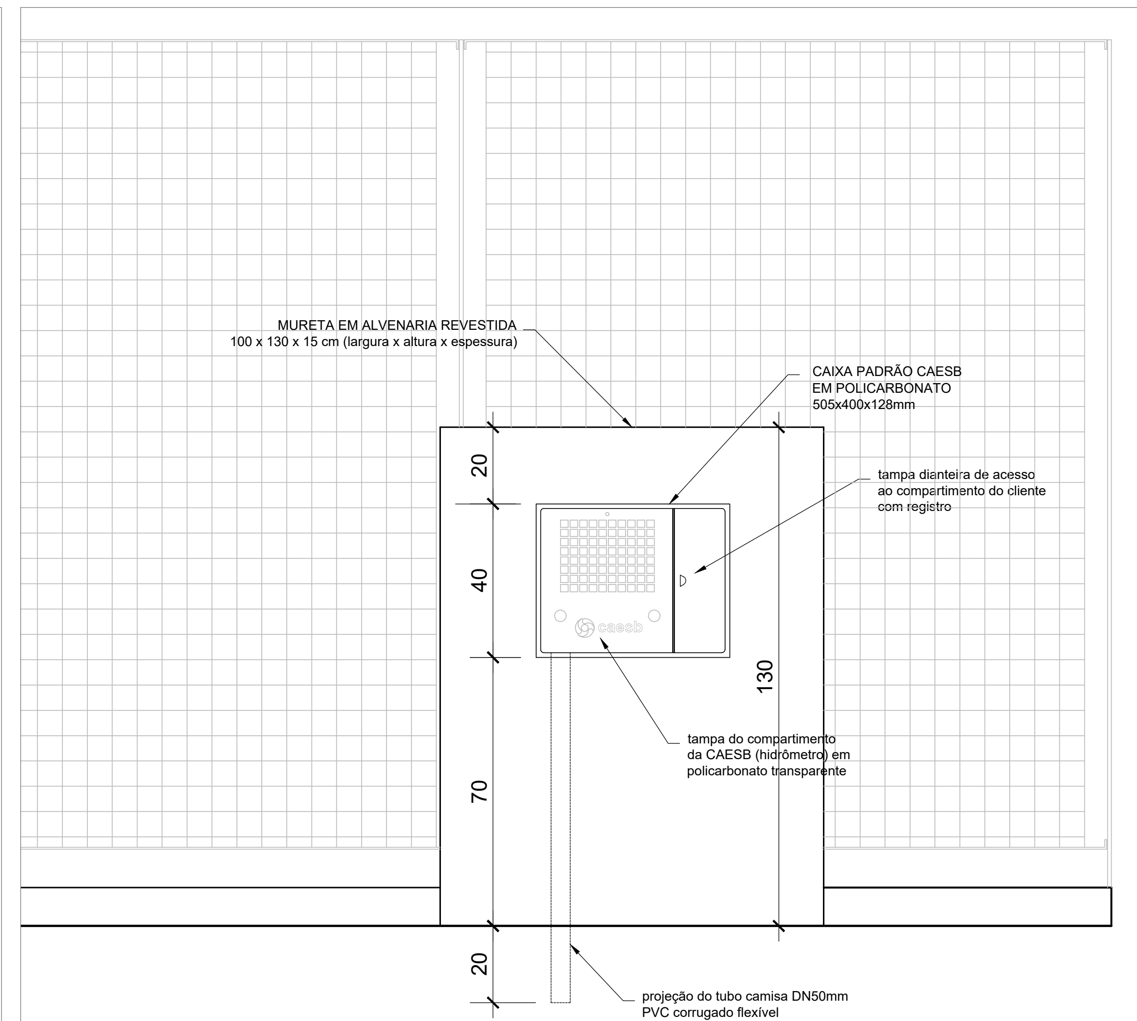
VISTA FRONTAL ESCALA:1/10
