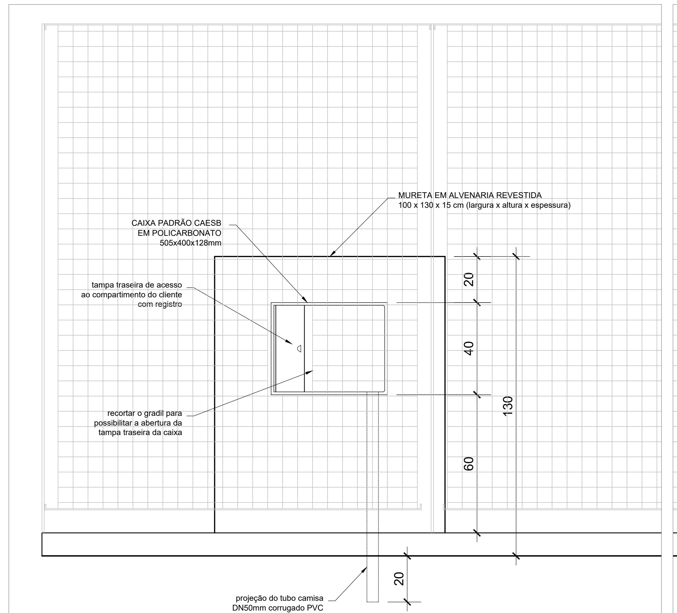
VISTA POSTERIOR ESCALA:1/10
