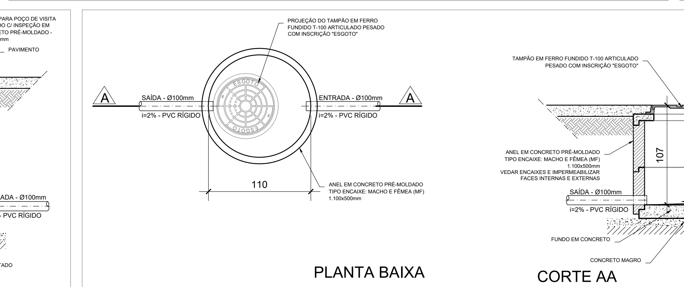
DETALHE DE CAIXA DE INSPEÇÃO P/ ESGOTO SANITÁRIO PROFUNDIDADE = 107cm ESCALA:1/25
