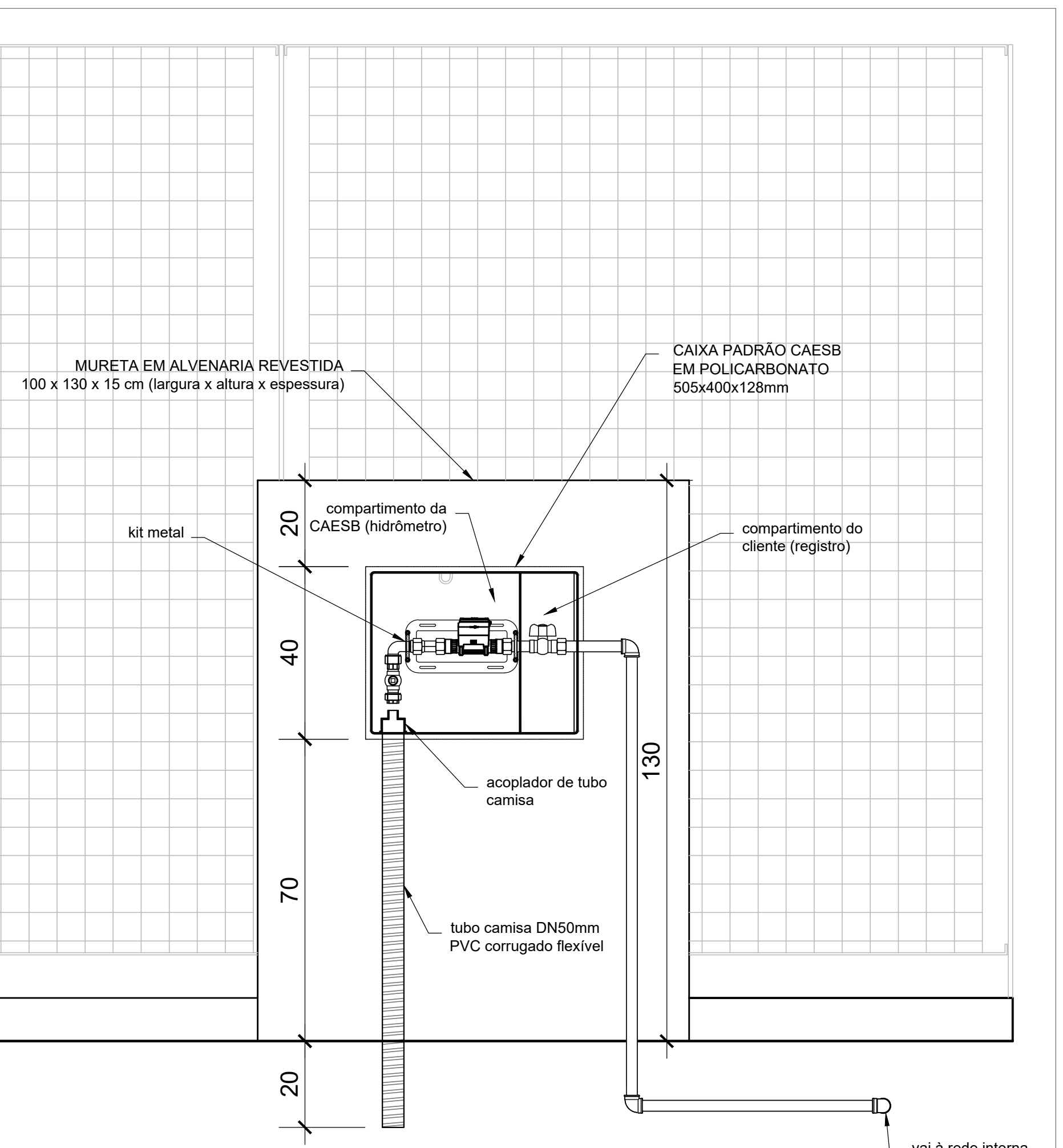
CORTE CC ESCALA:1/10
