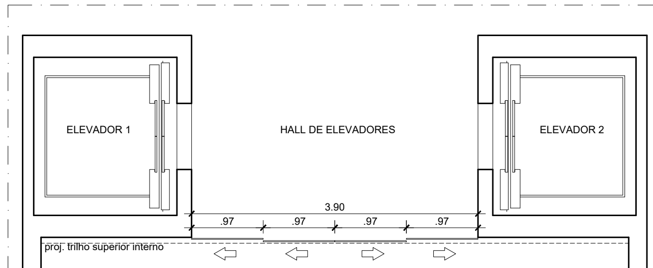
PLANTA. porta a instalar esc 1/50
