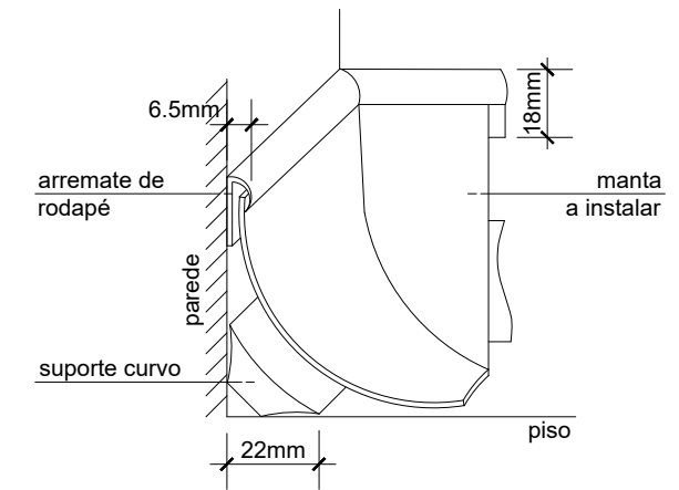
Rodapé curvo na própria manta h=10cm esc 1/2
