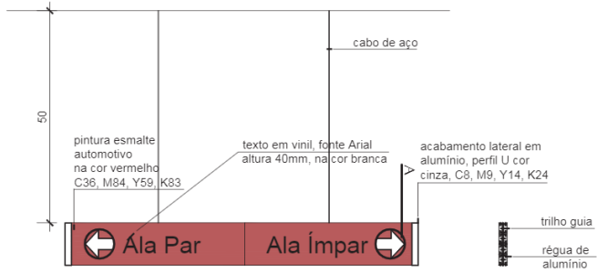
POP - PLACA DE ORIENTAÇÃO DE PAVIMENTO VISTA FRONTAL esc 1/10
