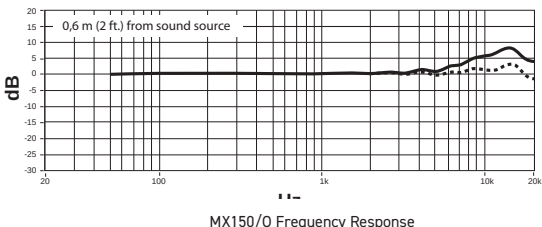
Boost Cap Normal Cap
