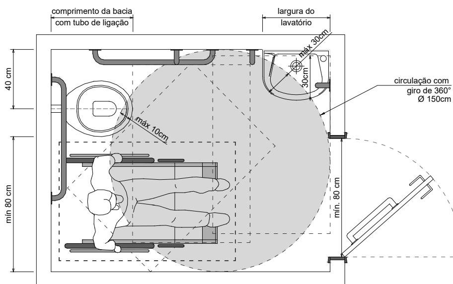
Figura 72 - Sanitário acessível (Cartilha de acessibilidade do Crea-SC)
