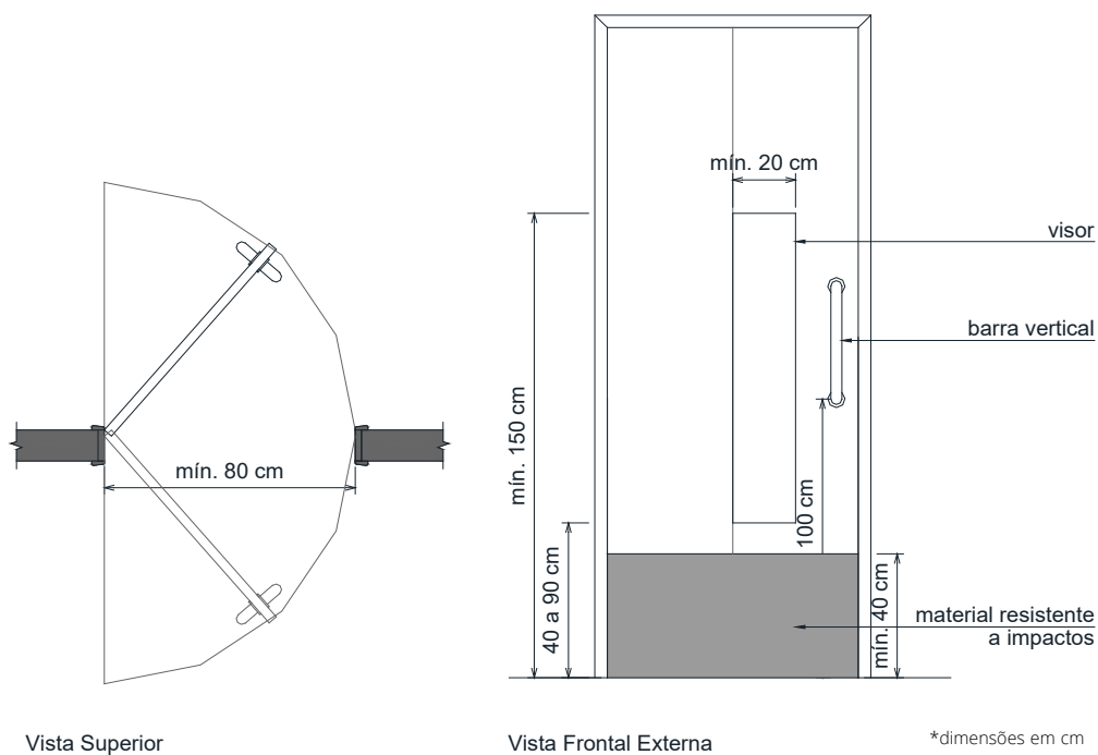
Figura 67 - Características das portas (Cartilha de acessibilidade do Crea-SC)
