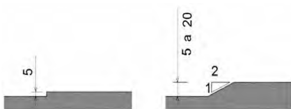
Figura 48 - Tratamento de desníveis até 20mm (Cartilha de acessibilidade do Crea-SC)
