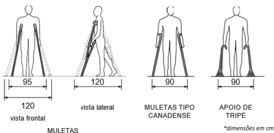
Figura 8 - Dimensões referenciais para deslocamento de pessoas com muletas (Cartilha de acessibilidade do Crea-SC)
