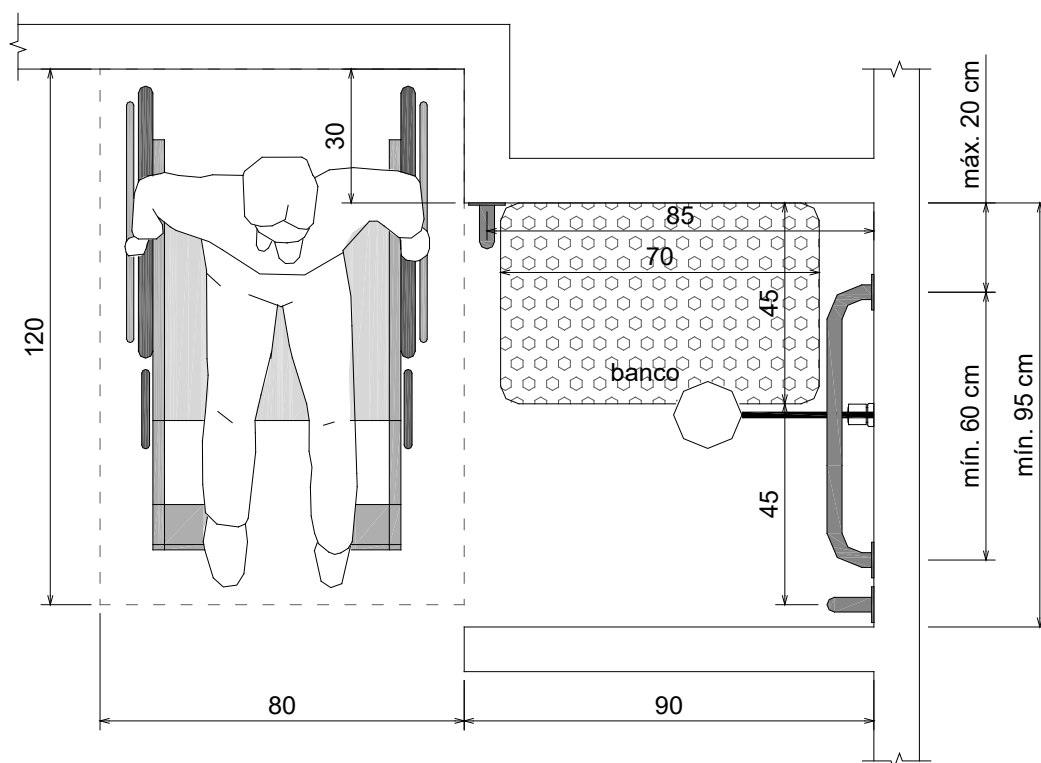
Figura 85 - Box para chuveiro acessível – vista superior (Cartilha de acessibilidade do Crea-SC)
