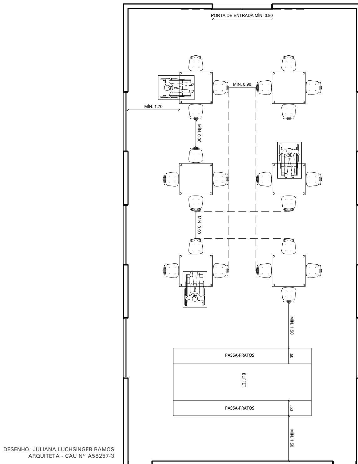
Figura 93 - Disposição mesas em restaurante, bares e similares – Vista Superior (Cartilha de acessibilidade nas empresas de alimentação Sebrae)
