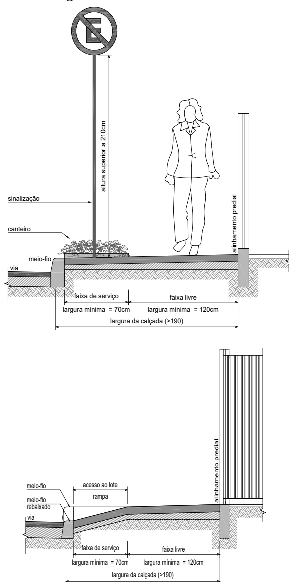
Figura 16 - Passeio com largura mínima (Cartilha de acessibilidade do Crea-SC)
