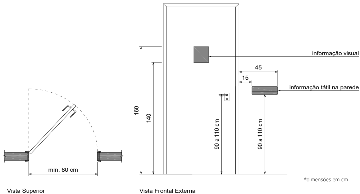
Figura 67 - Características das portas (Cartilha de acessibilidade do Crea-SC)
