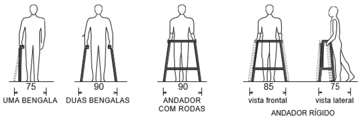
Figura 7 - Dimensões referenciais para deslocamento de pessoas com bengala e andador (Cartilha de acessibilidade do Crea-SC)
