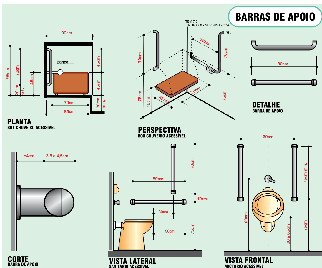
Figura 86 - Barras de apoio (Cartilha de acessibilidade da Prefeitura de Uberlândia)
