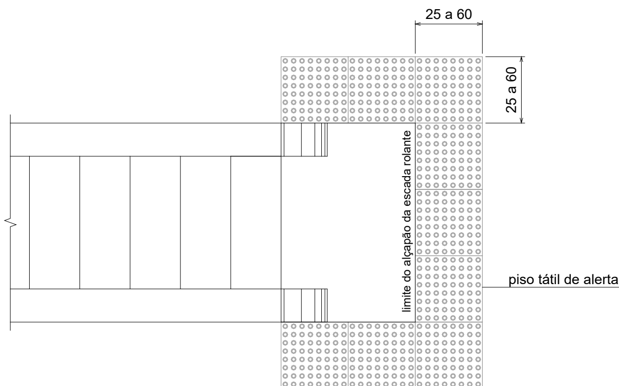
Figura 62 - Detalhes construtivos para elevador (Cartilha de acessibilidade do Crea-SC)
