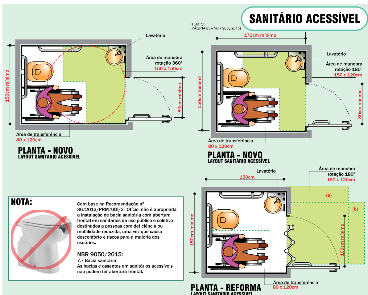
Figura 80 - Sanitário acessível (Cartilha de acessibilidade da Prefeitura de Uberlândia)
