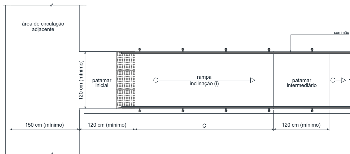
Figura 54 - Patamar de rampa – exemplo (Cartilha de acessibilidade do Crea-SC)
