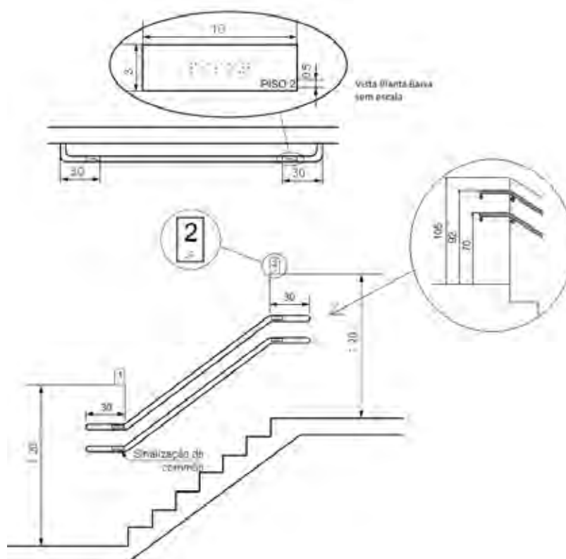
Figura 58 - Instalação de guarda-corpo e corrimão (Cartilha de acessibilidade do Creg-SC)
