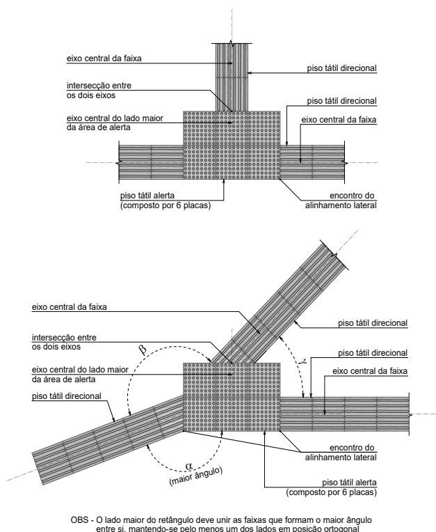
Figura 23 - Mudança de direção – encontro de duas faixas (Cartilha de acessibilidade do Crea-SC)
