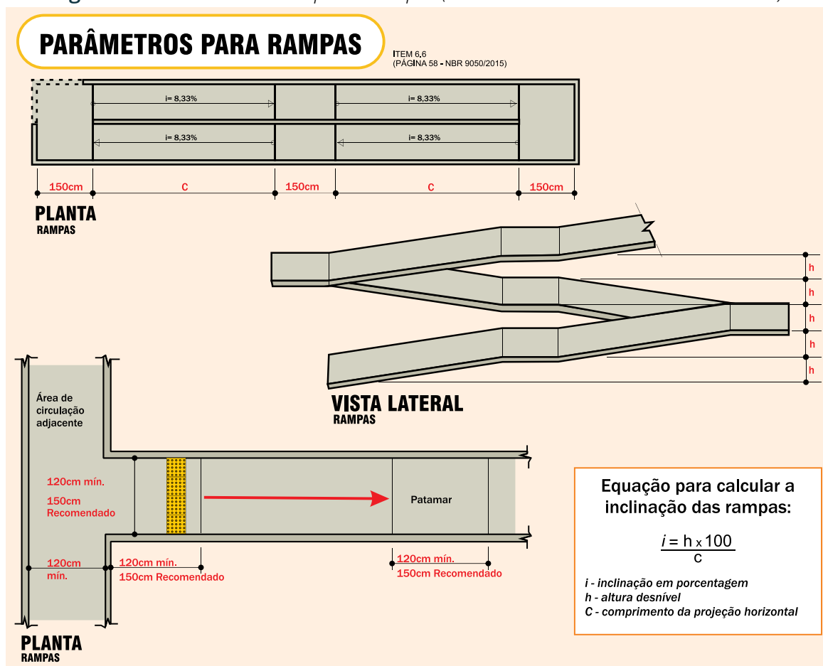
Figura 54 - Patamar de rampa – exemplo (Cartilha de acessibilidade do Crea-SC)
