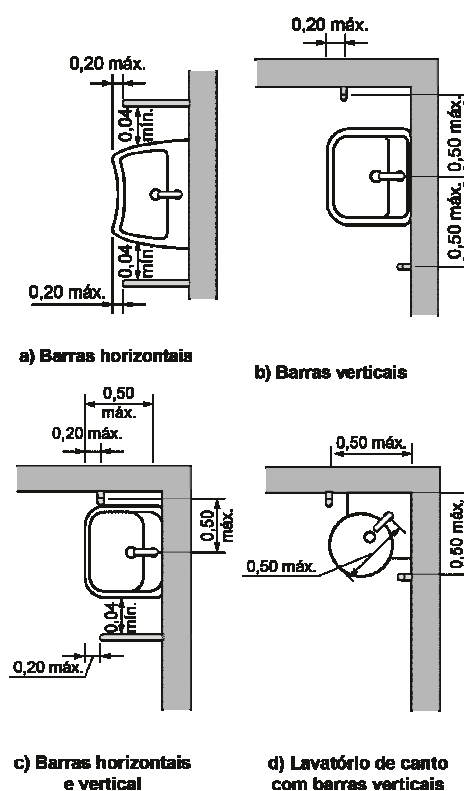
Figura 78 - Barras de apoio dos lavatórios (Nota Técnica 06/2016 do MPF)
