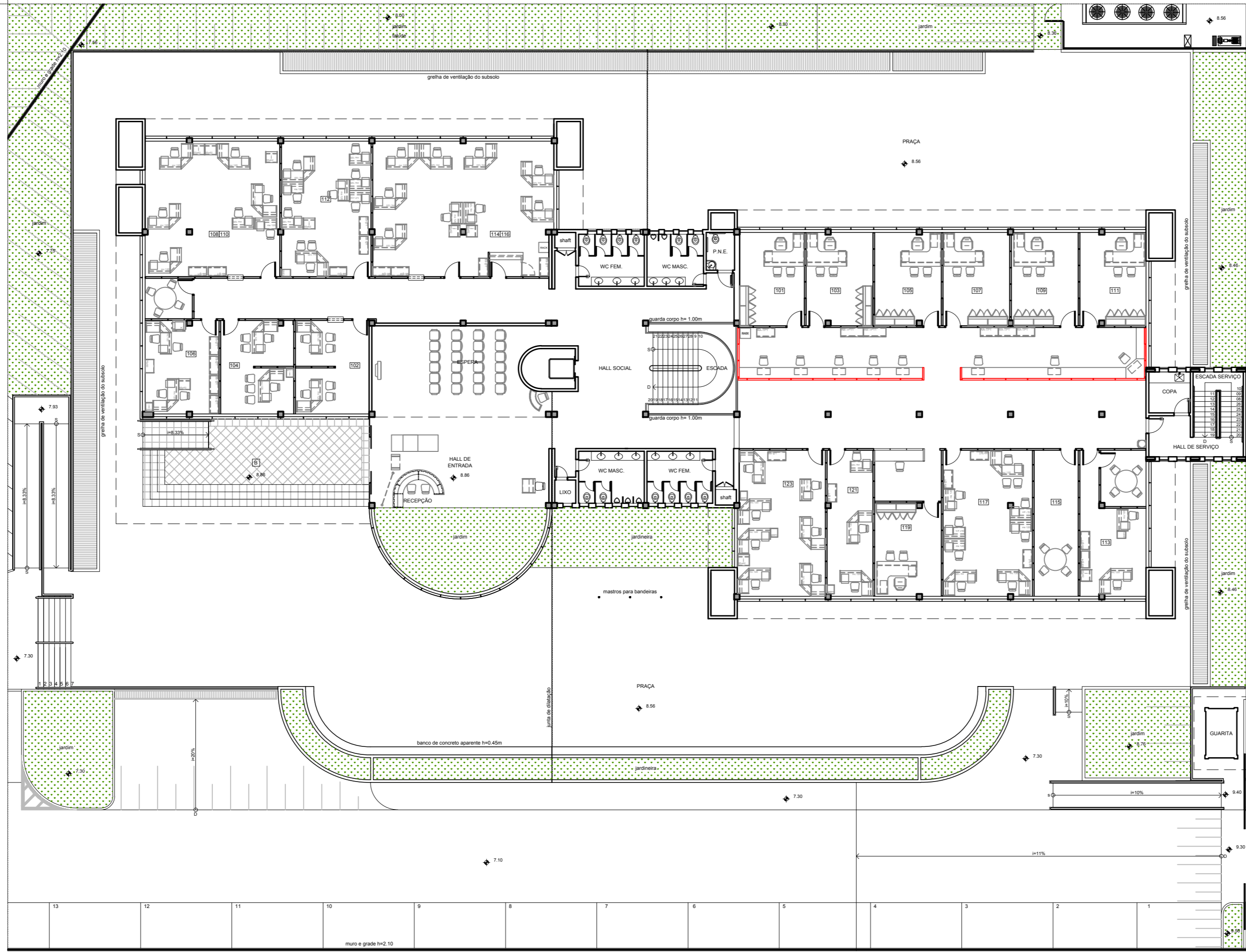
PLANTA BAIXA - TÉRREO esc 1/100
